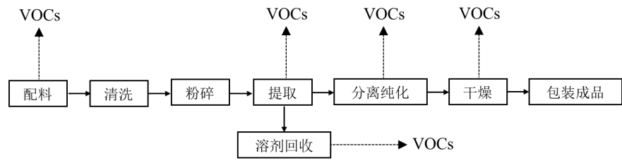
图 1-3 提取制药生产工艺与 VOCs 排放环节图
