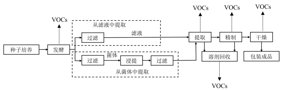
图 1-1 发酵制药生产工艺与 VOCs 排放环节图
