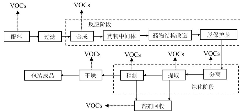
图 1-2 化学合成制药生产工艺与 VOCs 排放环节图
