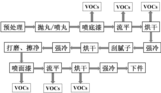
图 1-1 工程机械整机制造业生产工艺与 VOCs 排放环节示意图
