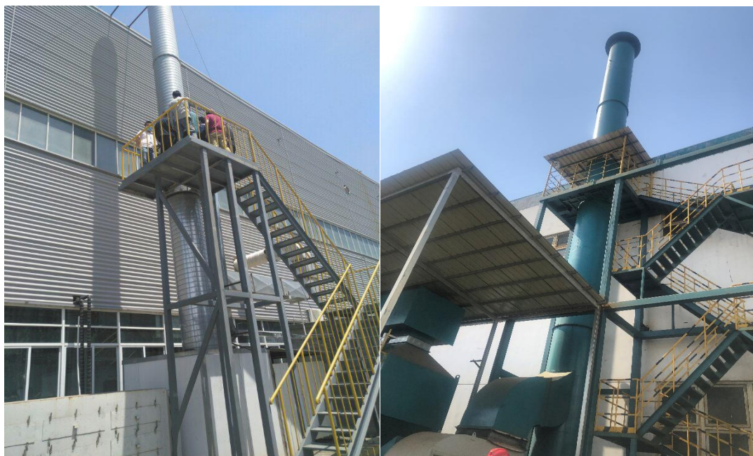
图 4-2 规范化的排污口示例一
