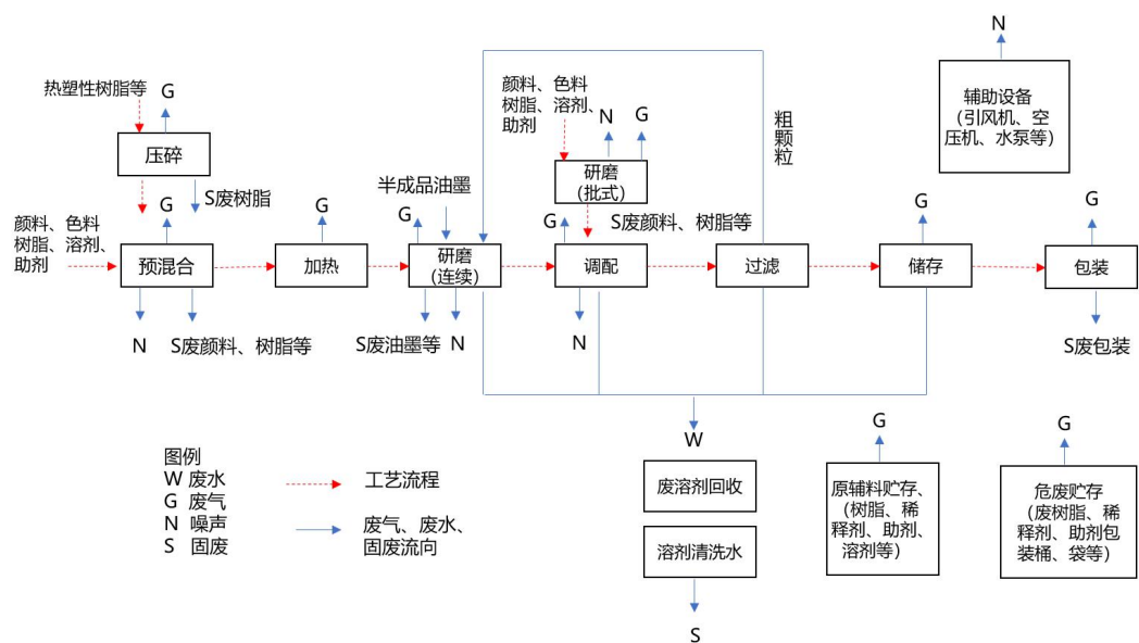
图 1-1 涂料、油墨及胶粘剂制造业生产工艺与污染物排放环节示意图
