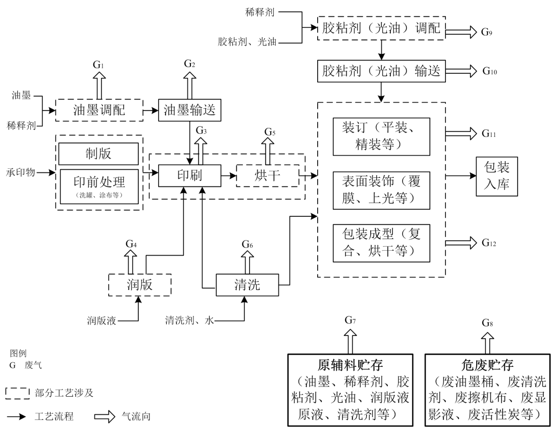
图 1 包装印刷行业生产工艺与 VOCs 排放环节示意图
