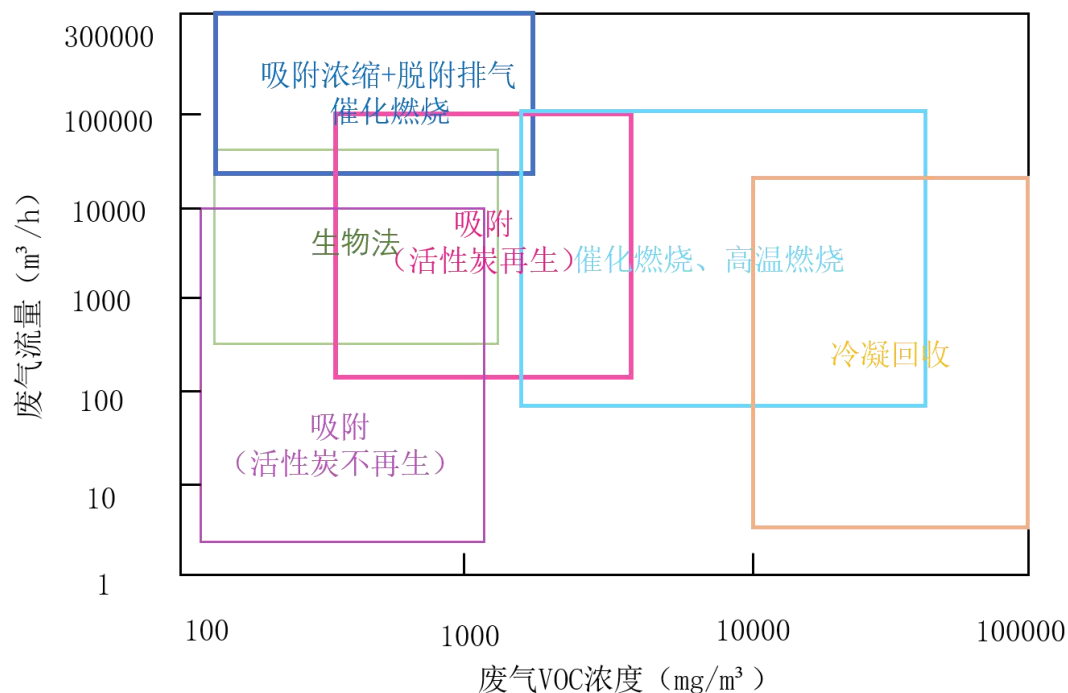
图 6 VOCs 治理技术适用范围（浓度、风量）
